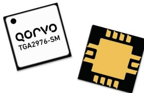
AC-QFN 4x4 mm 14L
