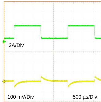
12 V_{IN} , 3.3 V_O , 0.5- to 3-A Step
