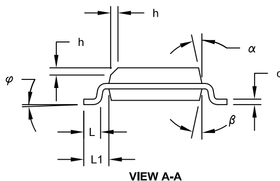
VIEW A-A
