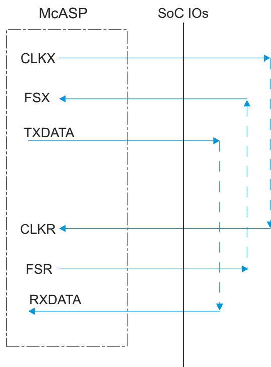
图 7-44. McASP1-8 COIFIO - ASYNC Mode
