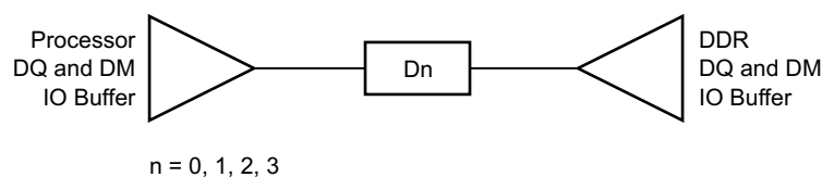
图 8-23. DQ/DM Topology
