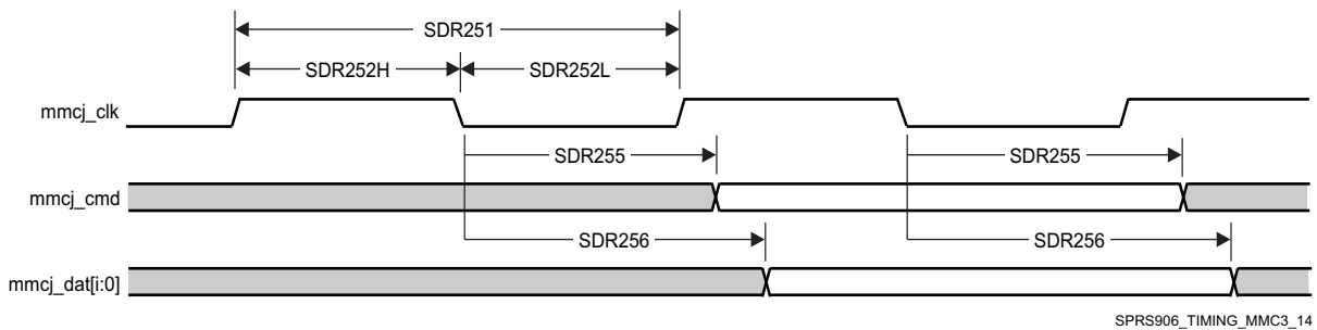
图 7-88. MMC/SD/SDIOj in - SDR25 - Transmitter Mode
