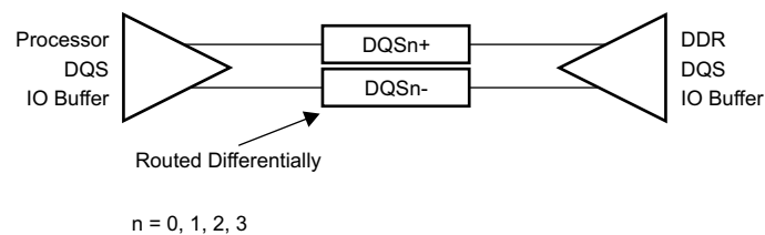
图 8-22. DQS Topology
