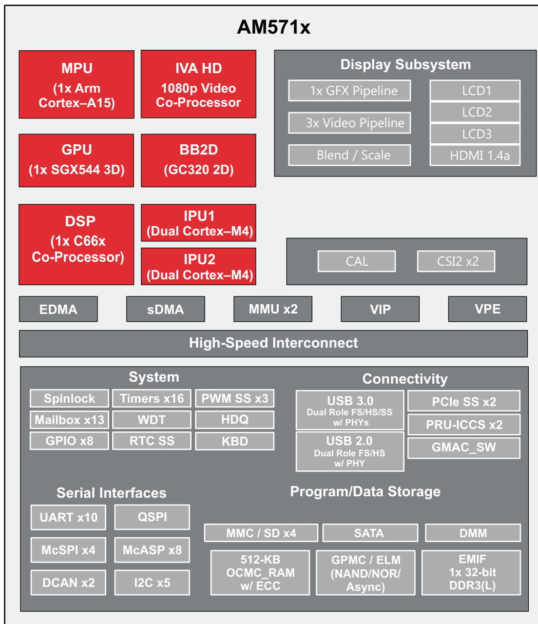
图 1-1. AM571x 框图
