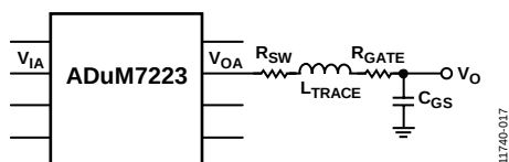
图17. N通道MOSFET栅极的RLC模型
