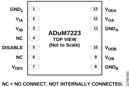
图3. 引脚配置
