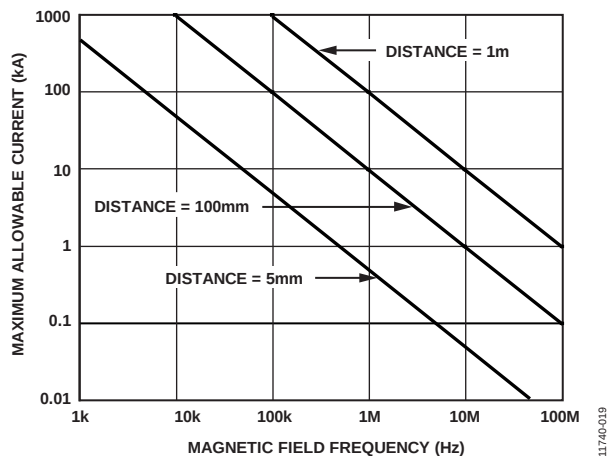
图19. 不同电流至ADuM7223距离下的最大允许电流
