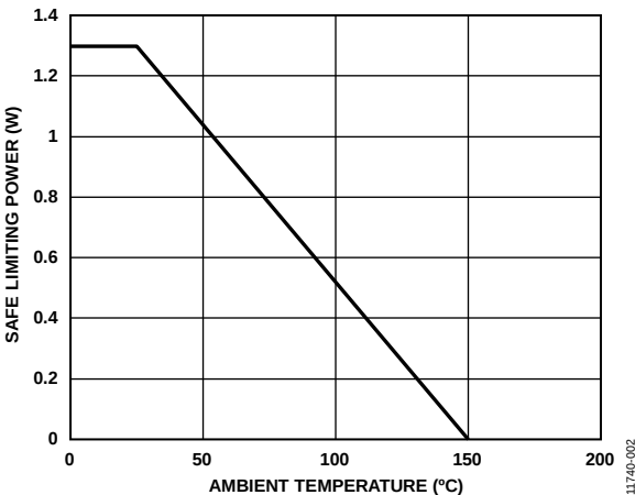
图2. 热减额曲线
