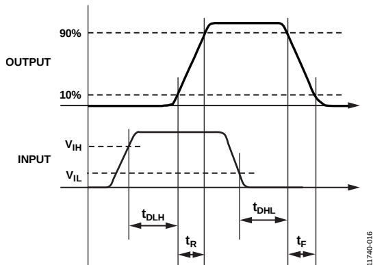
图16. 传播延迟参数
