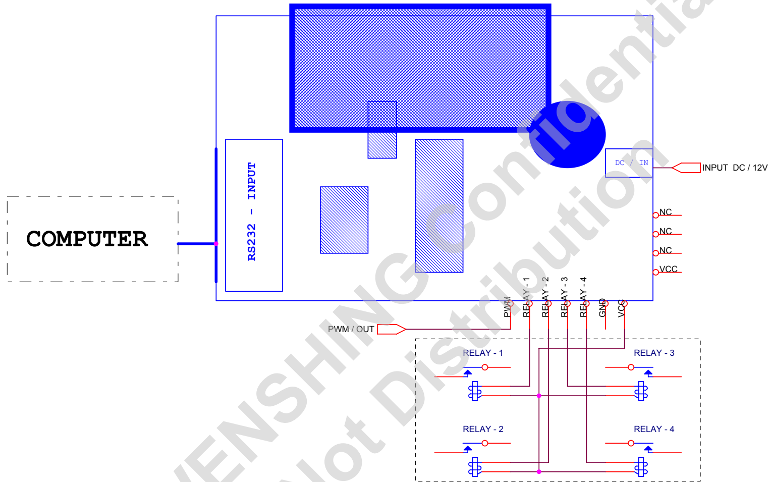
外接 RELAY 板
