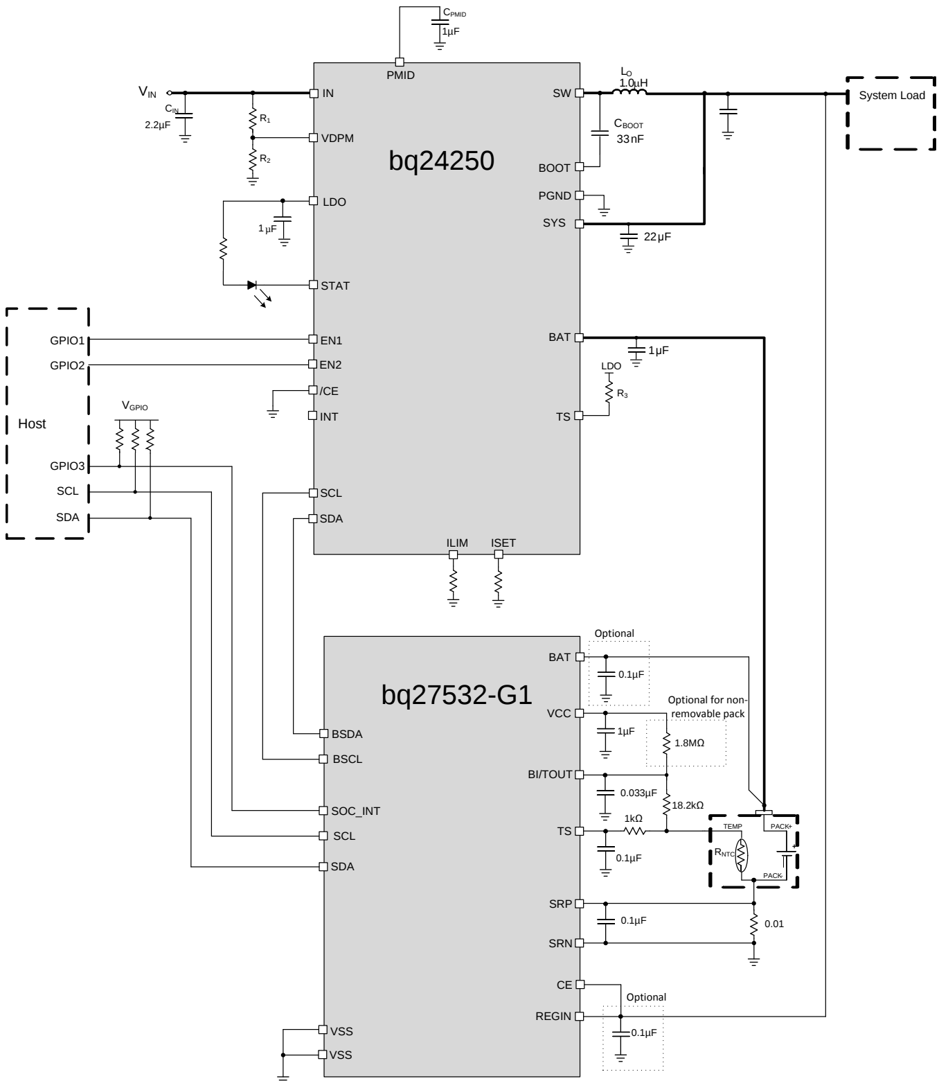
图 6. Schematic
