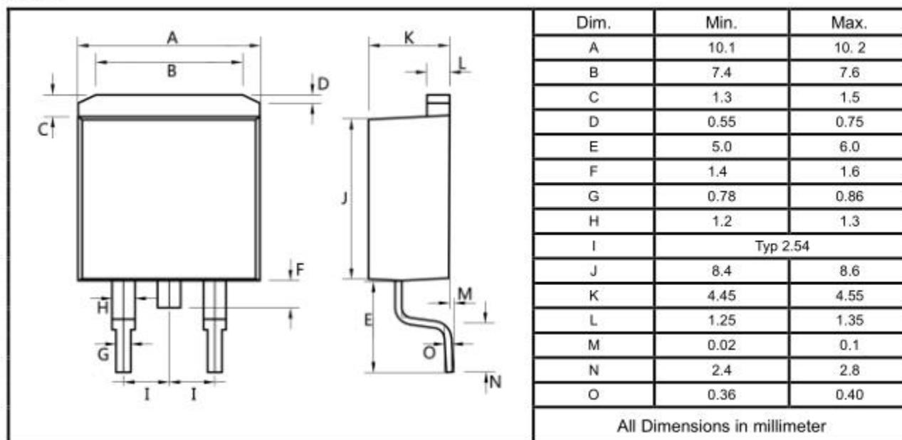
TO-263
