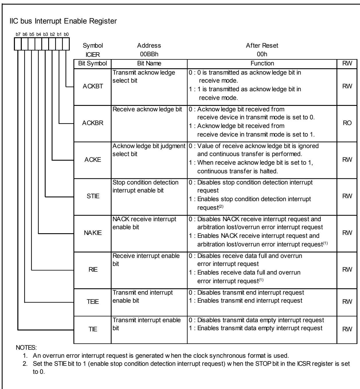
Figure 16.29 ICIER Register
