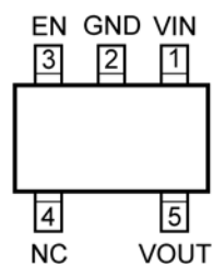
MIC5232-x.xYD5 TSOT-23-5 (D5)
