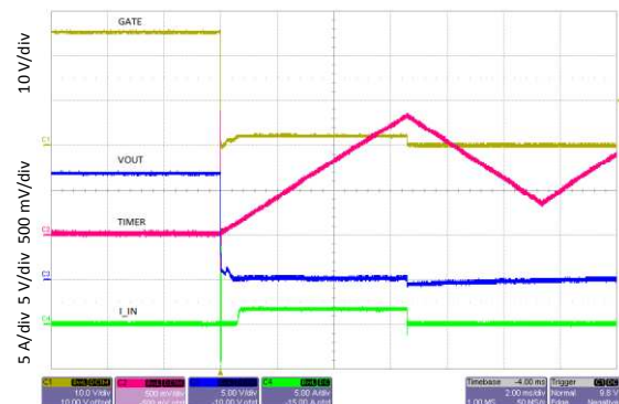
瞬态输出短路响应
