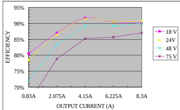
Vo=12 V
