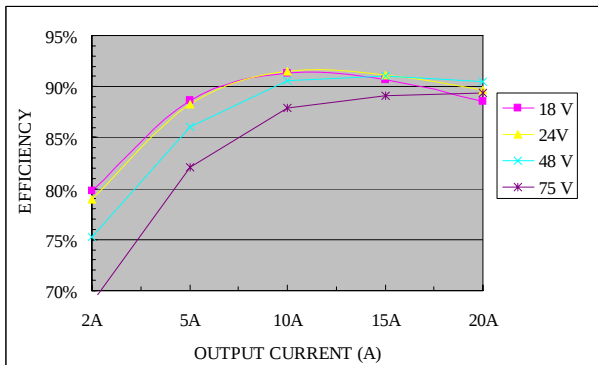
Vo=5.0 V
