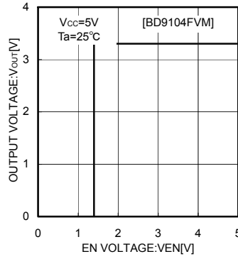
Fig.5 V EN -V OUT
