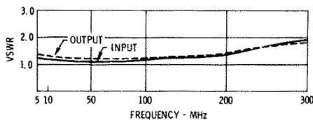
VSWR
