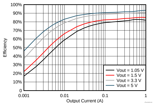
TPS561201 效率
