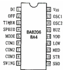
图 1 BA8206 BA4 的引脚说明
