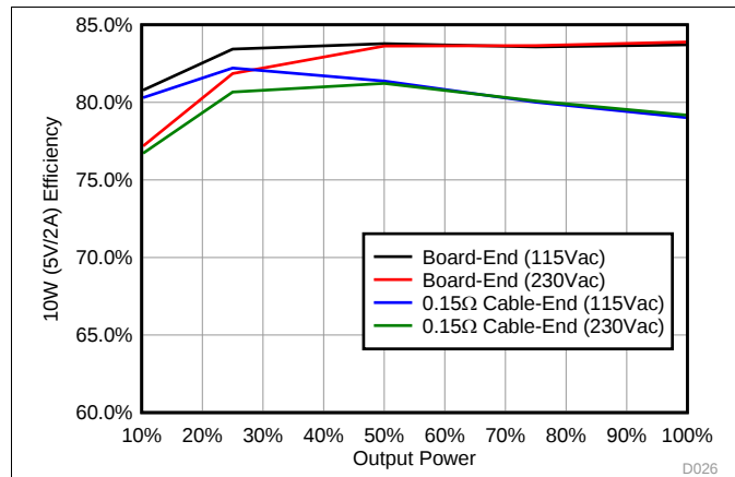
图 26. Efficiency
