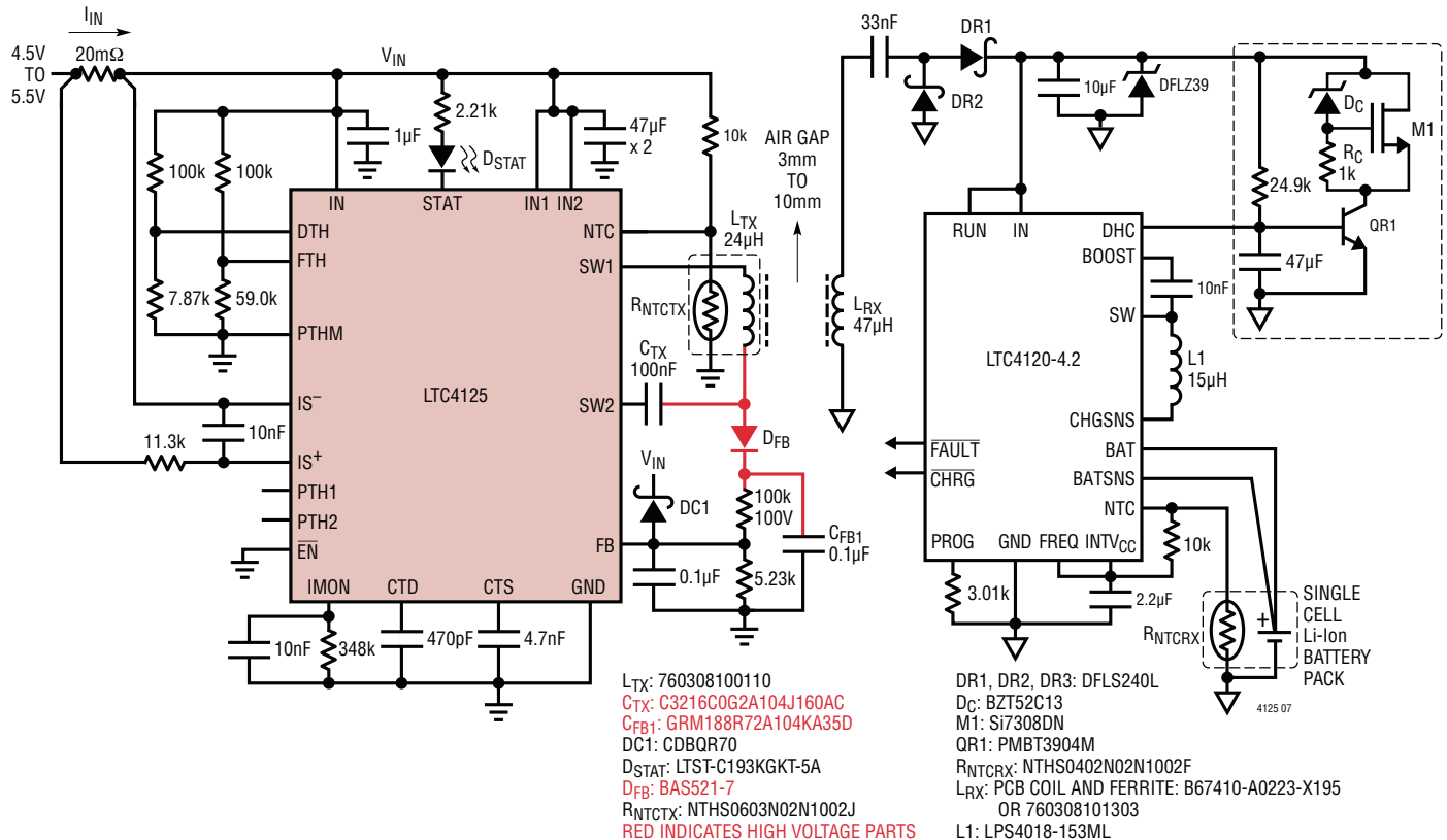
图 7：在一个把 LTC4120-4.2 作为接收器上的 400mA 单节锂离子电池充电器的无线功率系统中，LTC4125 在 103kHz 驱动一个 24µH 发送线圈，并采用 1.3A 输入电流门限，119kHz 频率限值及 41.5°C 发送线圈表面温度限值
