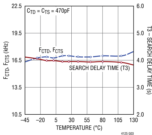
C TS 、C TD 引脚频率和搜索延迟 时间随温度的变化情况
