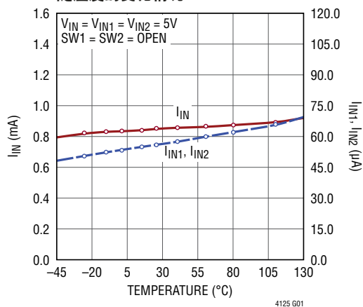
IN、IN1 和 IN2 上的电源静态电流 随温度的变化情况
