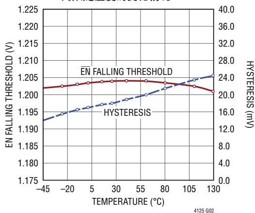
EN 门限随温度的变化情况
