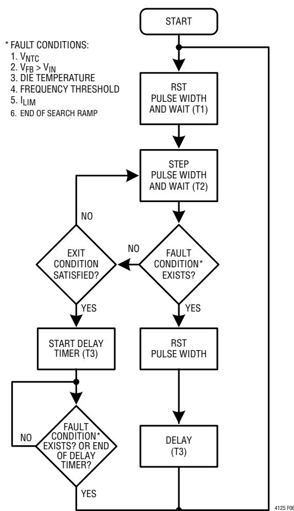
图 6：负载自动检测流程图
