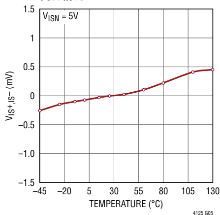
V IS+ 、IS- 检测放大器失调随温度的 变化情况
