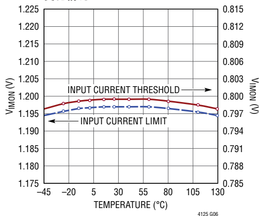
输入电流门限和限值随温度的 变化情况
