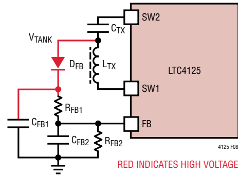
图 8：FB 引脚整流器和分压器
