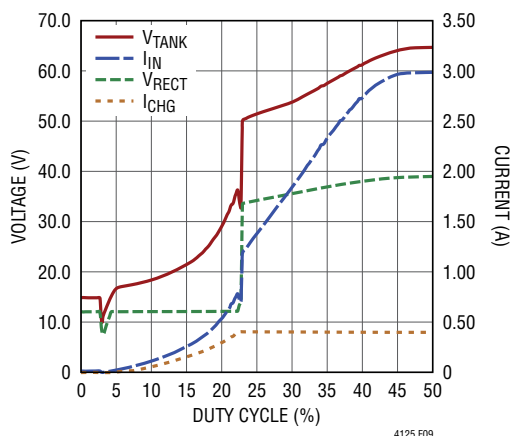
图 9： V_{TANK} 、 I_{IN} 、 V_{RECT} 和 I_{CHG} 与占空比的关系 (LTC4120 位于接收器，处于 CC 模式，间隔距离为 10mm)
