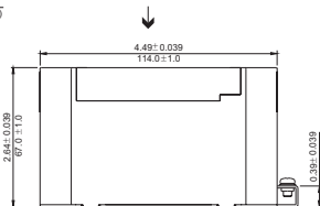
VIEW A.
