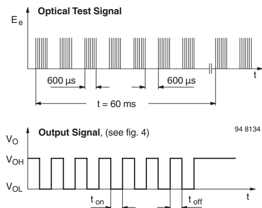
Fig. 3 - Output Function
