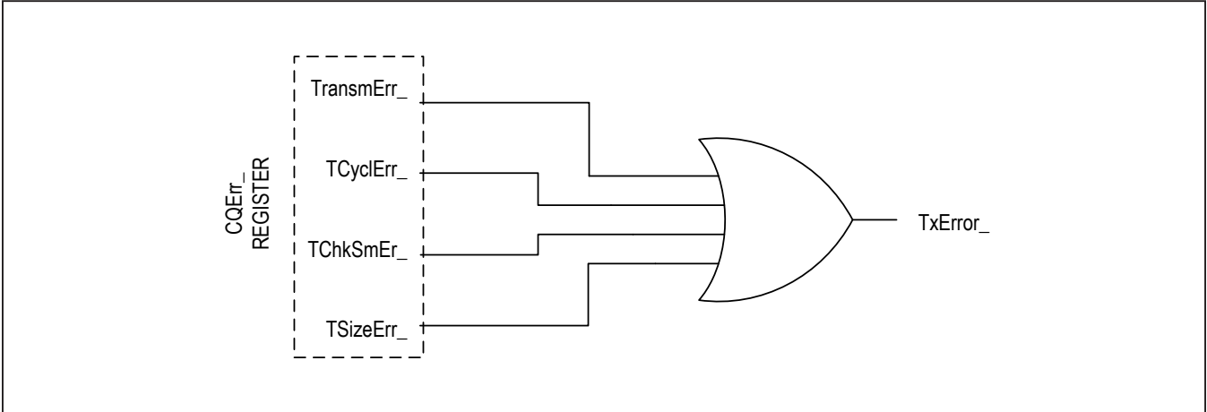
Figure 17. TxError_ Triggers
