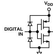
d. Digital Input
