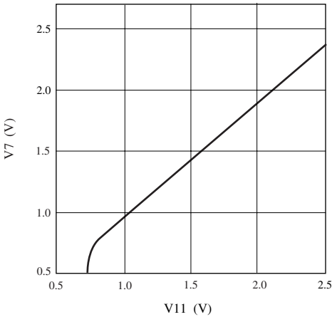
9. V_{CC} - V_{REF}
