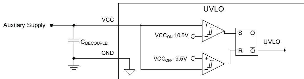
Figure 20. UVLO
