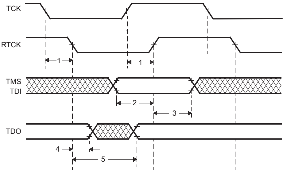
图 5-21. JTAG 时序
