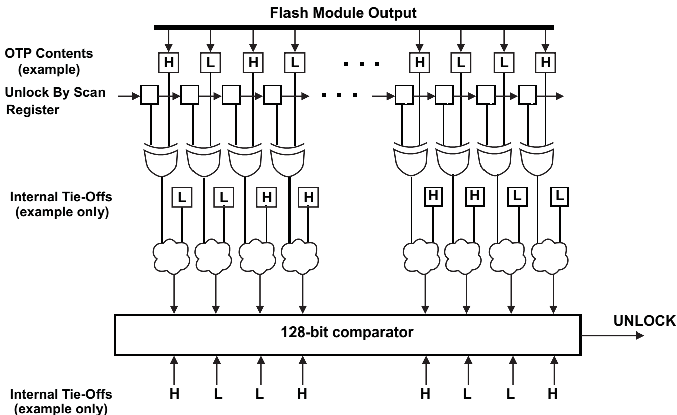
图 5-22. AJSM 解锁
