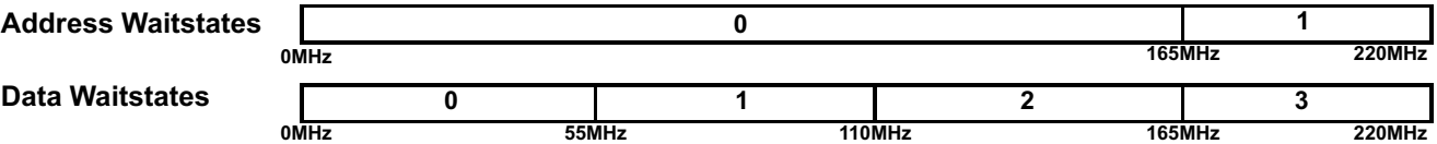
图 4-1. 等待状态机制
