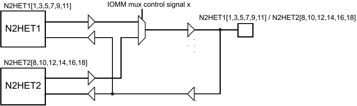
图 6-12. N2HET 监视
