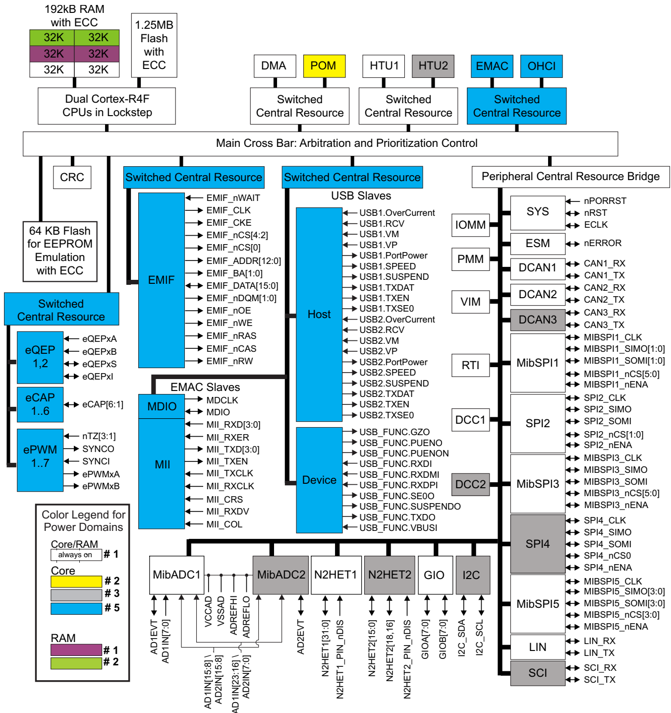
图 1-1. 功能方框图
