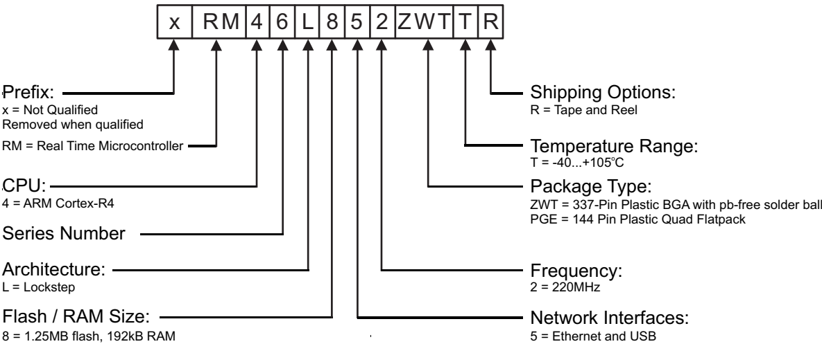
图 7-1. RM46L852 器件编号惯例
