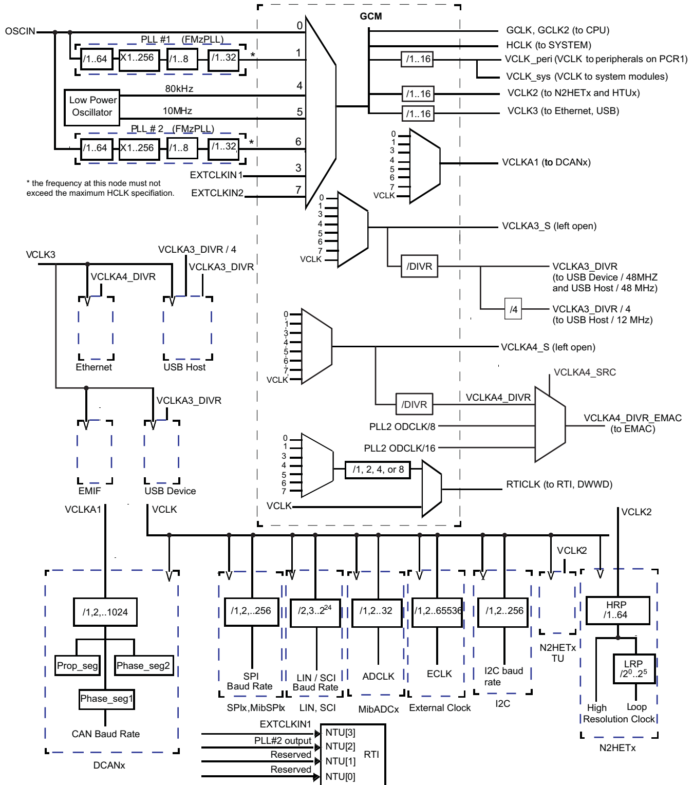
图 5-7. 器件时钟域
