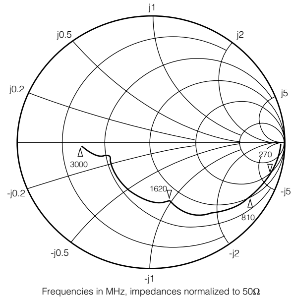
Fig. 5 Input Impedance
