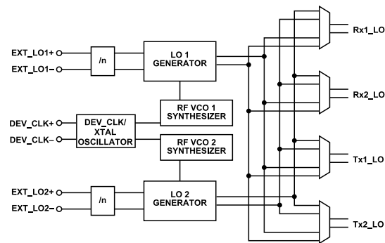
Figure 300. RF LO
