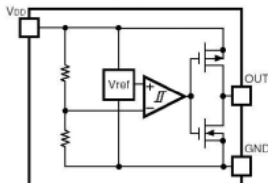
CMOS output
