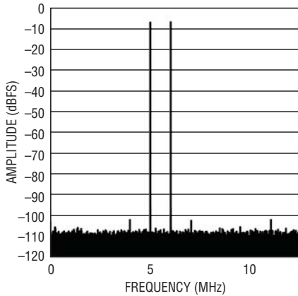
LTC2140-12: 64k Point 2-Tone FFT, f_{IN} = 69\text{MHz} , 70\text{MHz} , -7\text{dBFS} , 25\text{Mps}
