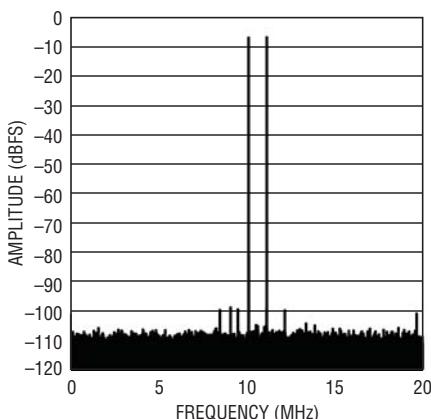
LTC2141-12: 64k Point 2-Tone FFT, f_{IN} = 69\text{MHz} , 70\text{MHz} , -7\text{dBFS} , 40\text{Msps}
