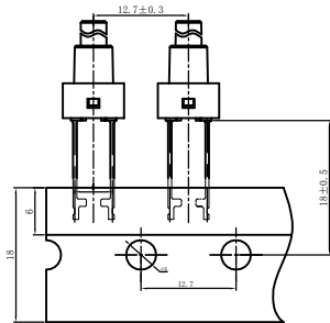
图1 编带图
