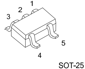
SOT-25
