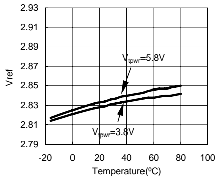
Vref - Temperature@Ivref=0mA
