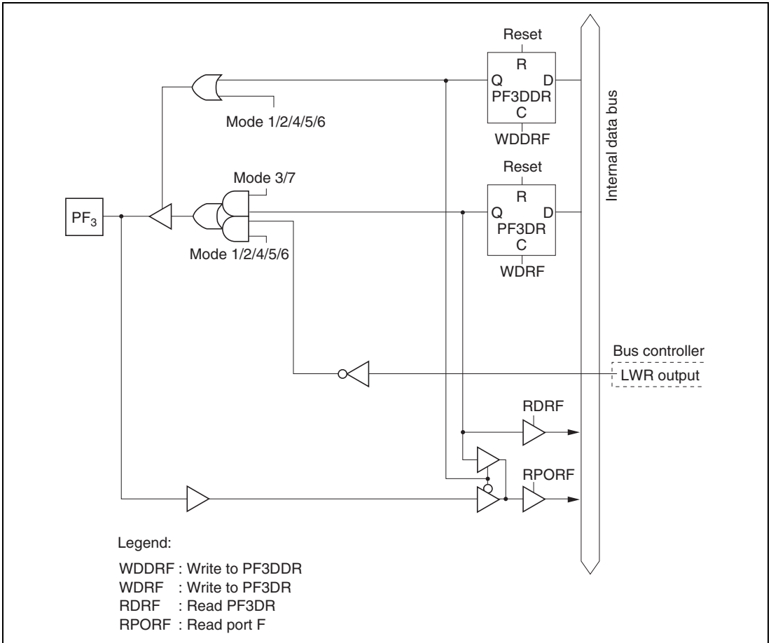
Figure C.12 (d) Port F Block Diagram (Pin PF 3 )
