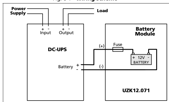
Fig. 8-1 Wiring scheme
