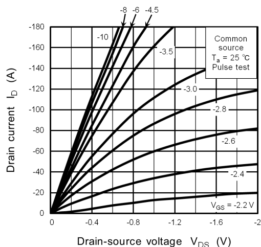
Fig. 8.2 I_D - V_{DS}
