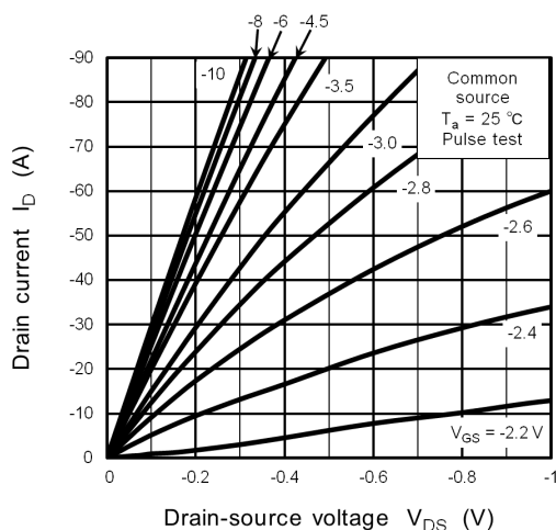
Fig. 8.1 I_D - V_{DS}
