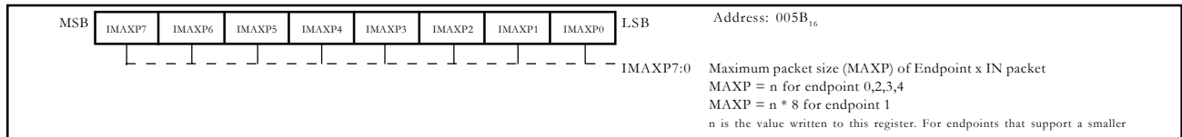
Fig. 1.66. USB Endpoint x IN MAXP Register (IN_MAXP)
