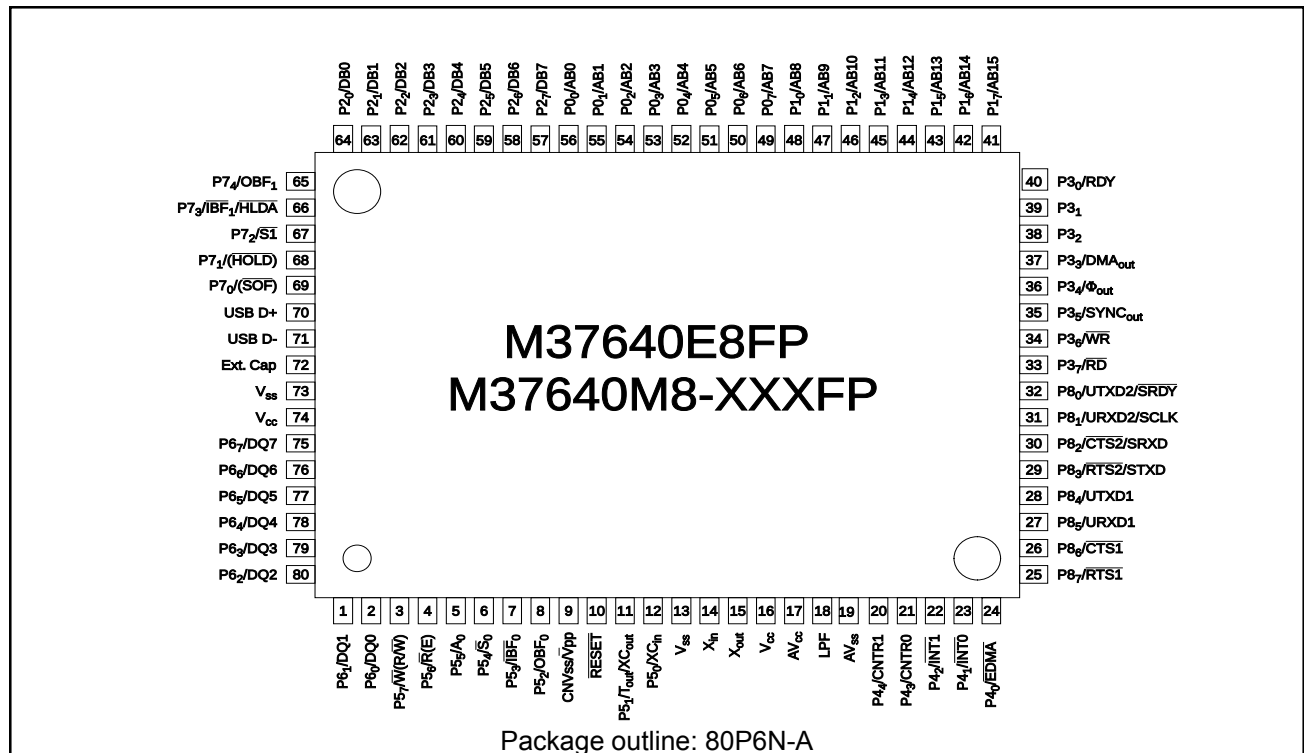
Fig. 1.1. Pin Layout
