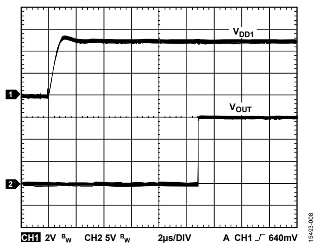
图8. 典型 V_{DD1} 延迟至输出波形, V_{IN} = V_{DD1}
