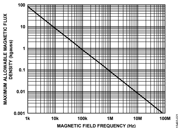
图24. 最大允许外部磁通密度
