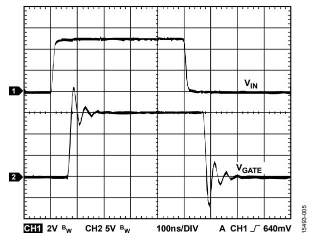
图5. ADuM4120 V_{IN} 至 V_{GATE} 波形, 2 nF 负载, 0 \Omega 串联栅极电阻, V_{DD2} = 15\text{ V}
