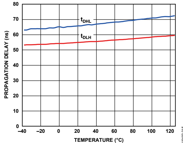
图15. ADuM4120 传播延迟与温度的关系, 2\text{ nF} 负载
