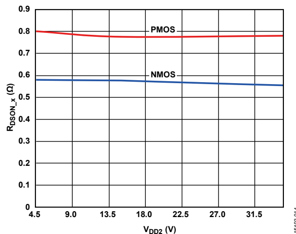
图14. R_{DS(on)} 与 V_{DD2} 的关系
