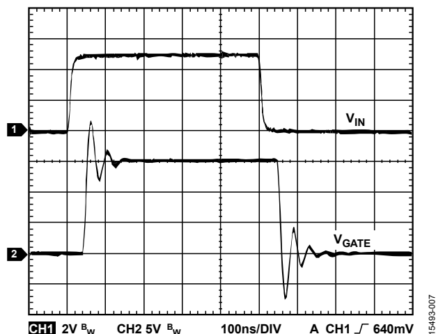
图7. ADuM4120-1 V_{IN} 至 V_{GATE} 波形, 2 nF 负载, 0 \Omega 串联栅极电阻, V_{DD2} = 15\text{ V}
