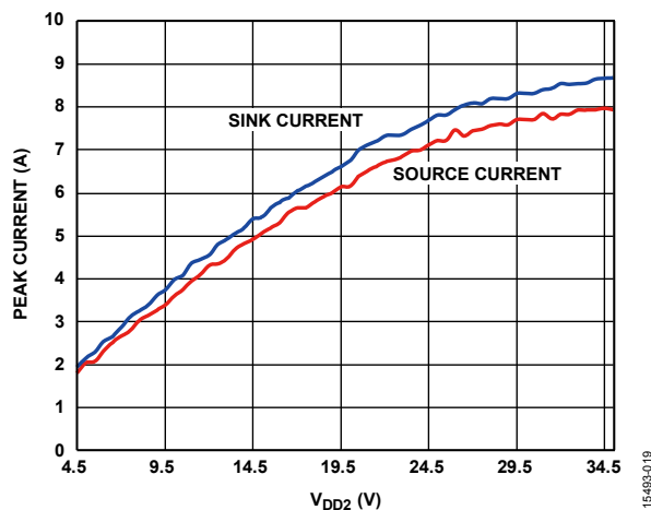
图19. 峰值电流与 V_{DD2} 的关系, 2 \Omega 电阻
