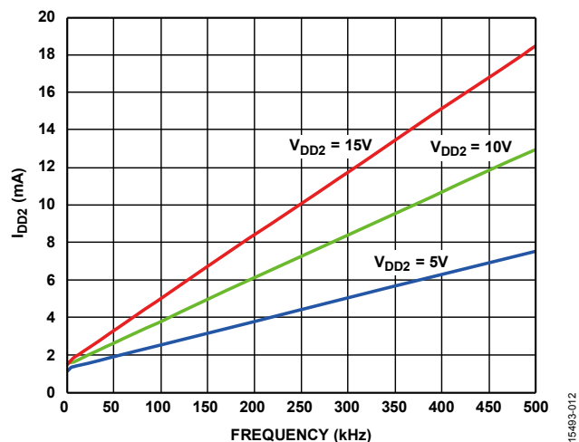
图12. I_{DD2} 与开关频率的关系, 2\text{ nF} 负载
