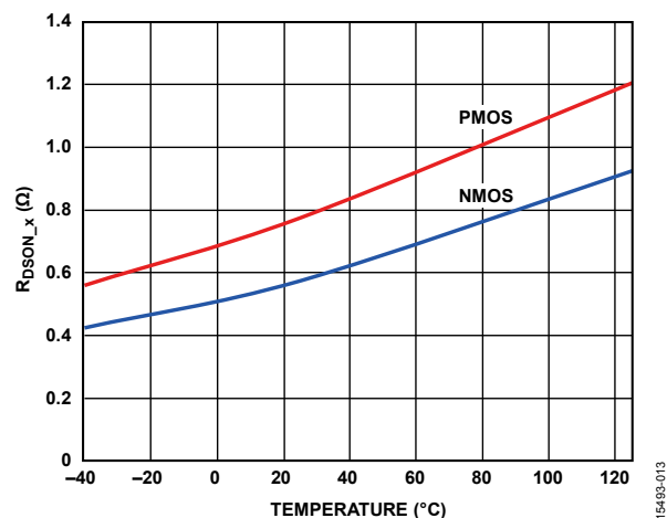
图13. R_{DS(on)} 与温度的关系
