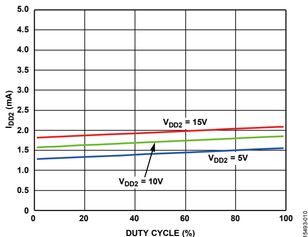
图10. I_{DD2} 与占空比的关系, V_{DD1} = 5V , f_{SW} = 10\text{ kHz} , 2\text{ nF} 负载
