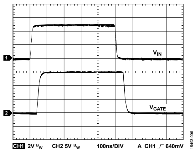
图5. ADuM4120 V_{IN} 至 V_{GATE} 波形, 2 nF 负载, 0 \Omega 串联栅极电阻, V_{DD2} = 15\text{ V}
