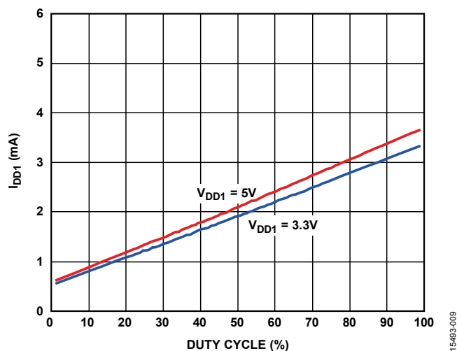
图9. I_{DD1} 与占空比的关系, f_{SW} = 10\text{ kHz}
