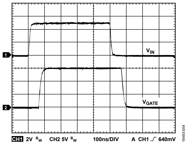
图4. ADuM4120 V_{IN} 至栅极电压( V_{GATE} )波形, 2 nF 负载, 5 \Omega 串联栅极电阻, V_{DD2} = 15\text{ V}
