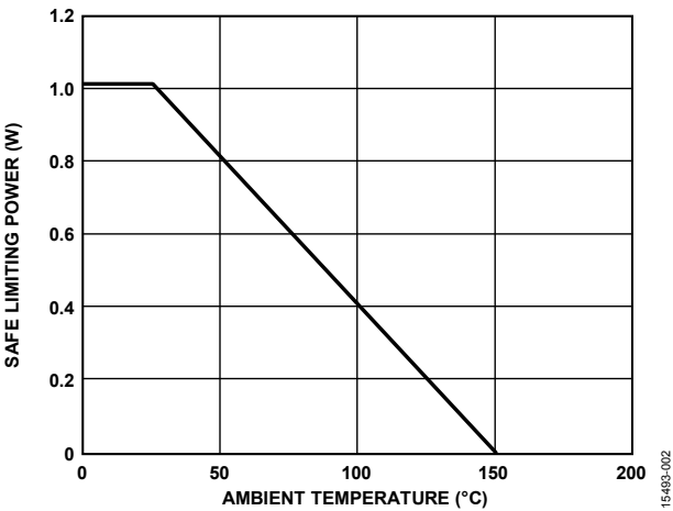
图 2. ADuM4120/ADuM4120-1 热减额曲线, 依据 DIN V VDE V 0884-10 获得的安全限值与壳温的关系
