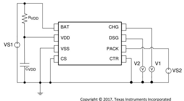
图 9-2. Test Circuit 2
