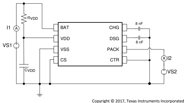
图 9-1. Test Circuit 1
