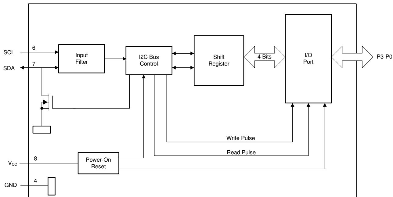
图 8-1. Logic Diagram
