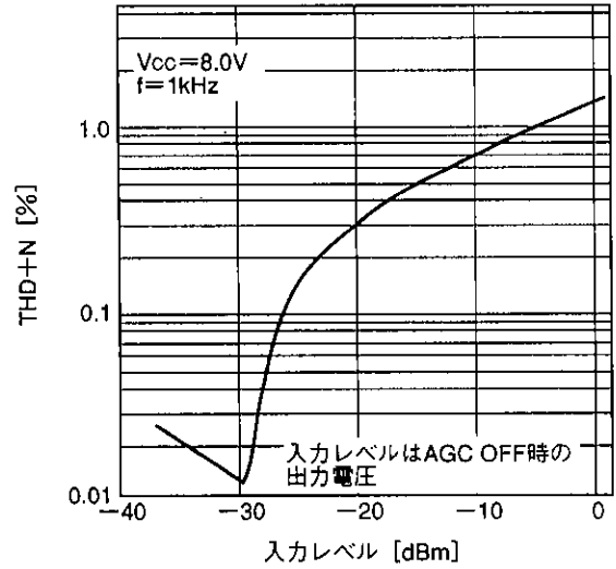
AGC全高調波歪率
