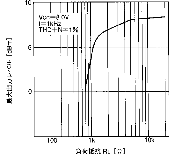
MIX Amp負荷特性
