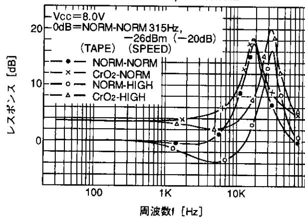
REC EQ Amp周波数特性
