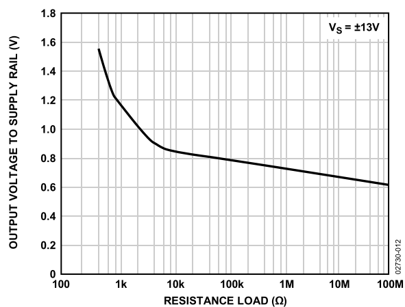
图12. 输出电压至供电轨与阻性负载的关系
