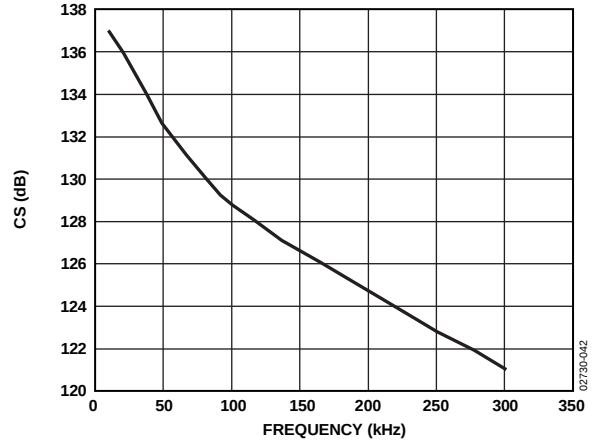
图42. AD8620通道隔离图
