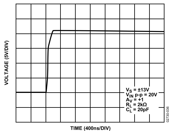
图36. 正压摆率( G = +1 )
