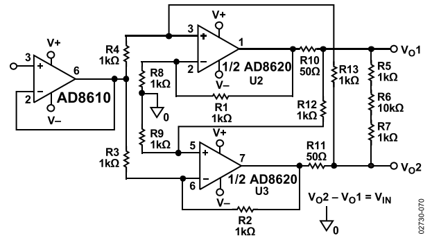
图70. 差分驱动器
