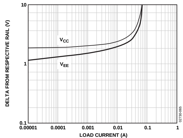
图65. OPA627相对于 \pm 15\text{ V} 的压差与负载电流的关系
