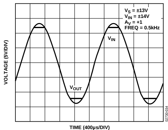
图34. 无相位反转
