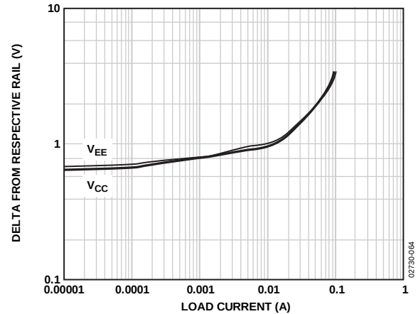
图64. AD8610/AD8620相对于 \pm 13\text{ V} 的压差与负载电流的关系
