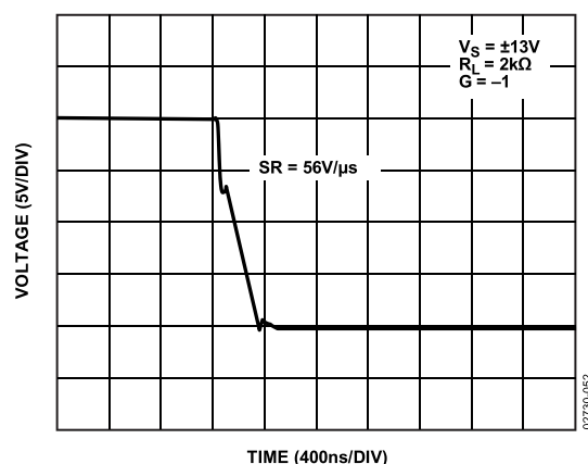
图52. -1的单位增益下OPA627的负压摆率
