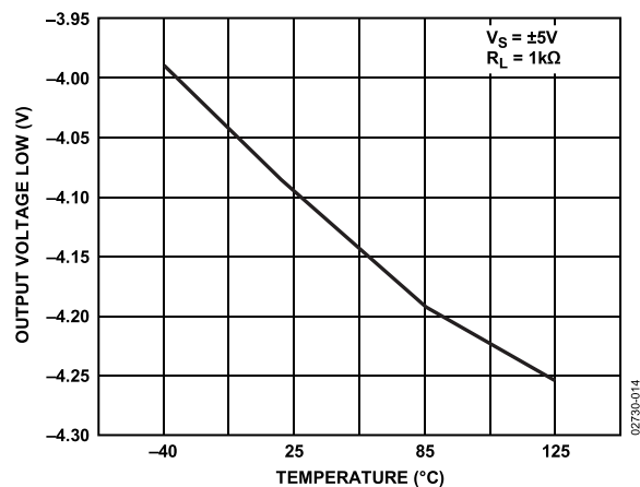
图14. 低输出电压低与温度的关系
