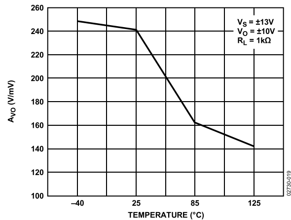
图19. A_{VO} 与温度的关系
