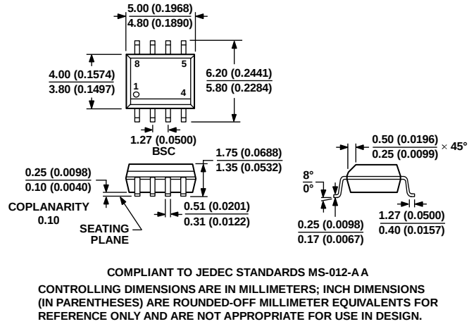
图72. 8引脚标准小型封装[SOIC_N]窄体(R-8) 图示尺寸单位: mm和(inch)
