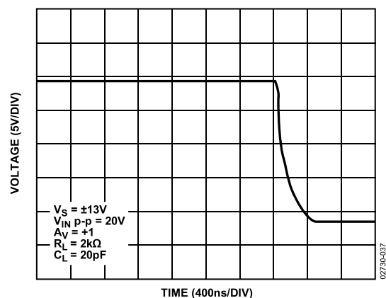
图37. 负压摆率( G = +1 )
