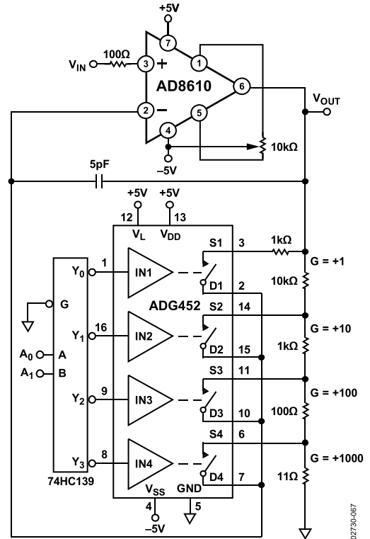
图67. 高精度PGA
