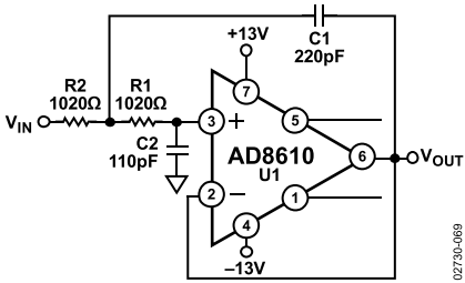
图69. 二阶低通滤波器
