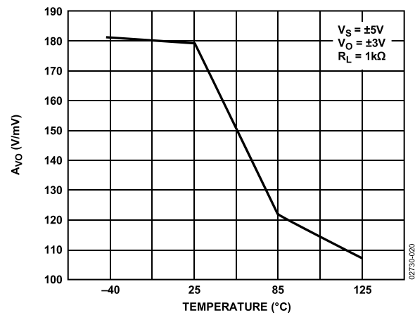
图20. A_{VO} 与温度的关系
