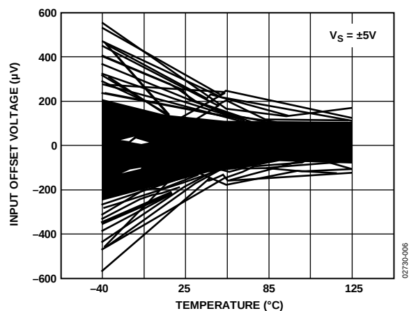
图6. \pm 5V 时输入失调电压与温度的关系(300个放大器)
