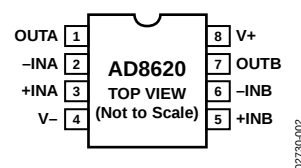
图2. 8引脚SOIC_N
