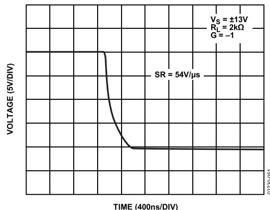
图51. -1的单位增益下AD8610/AD8620的负压摆率
