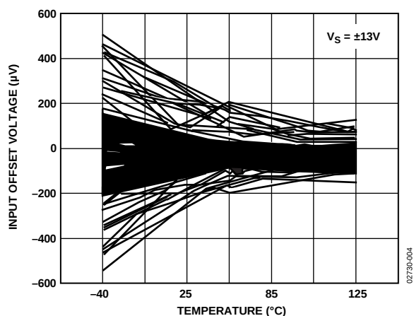
图4. \pm 13V 时输入失调电压与温度的关系(300个放大器)
