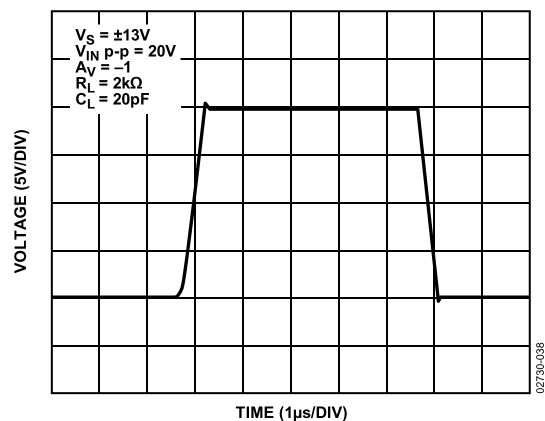
图38. 大信号瞬态响应( G = -1 )
