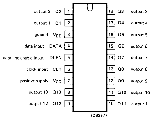
Fig. 2 Pinning diagram.
