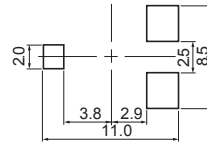
LAND PATTERNS (mm) 推奨ランド寸法
