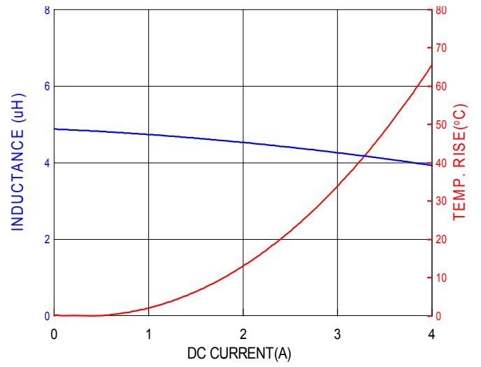
PIT07012-4R7M
