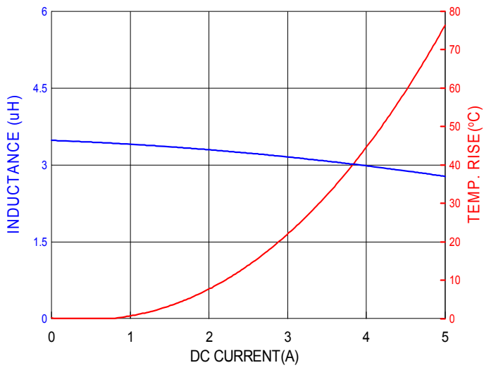
PIT07012-3R3M
