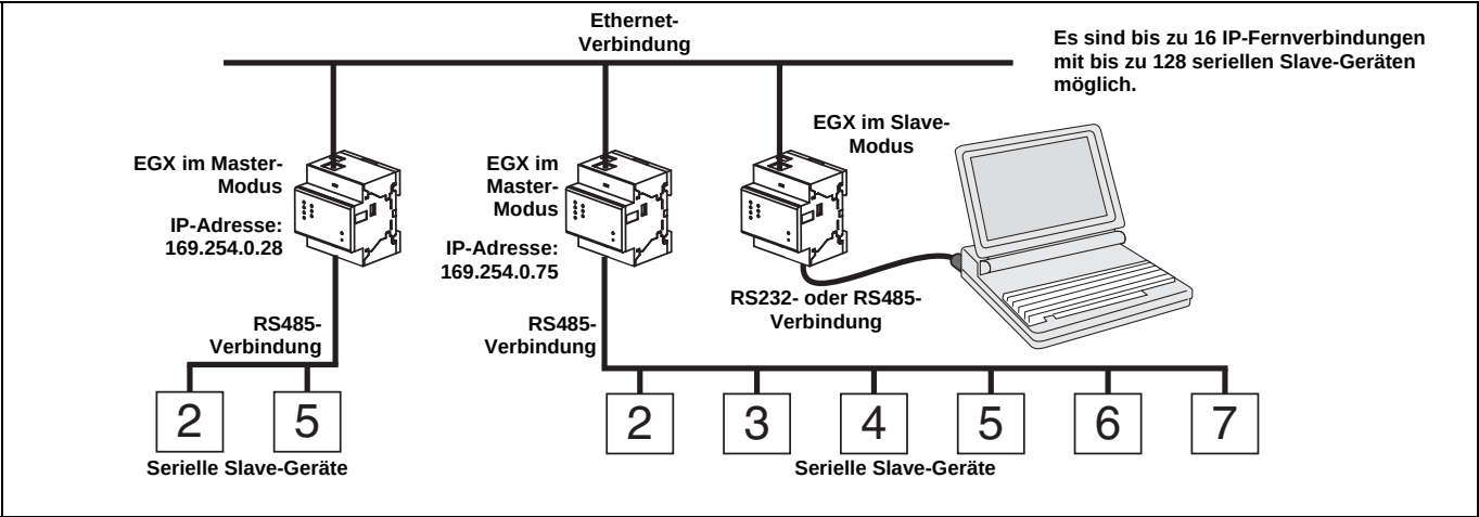
Abbildung 6: Slave-Modus-Topologie
