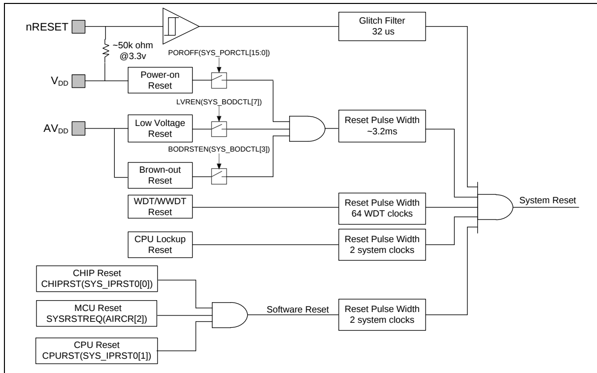
图 6.3-1 系统复位源
