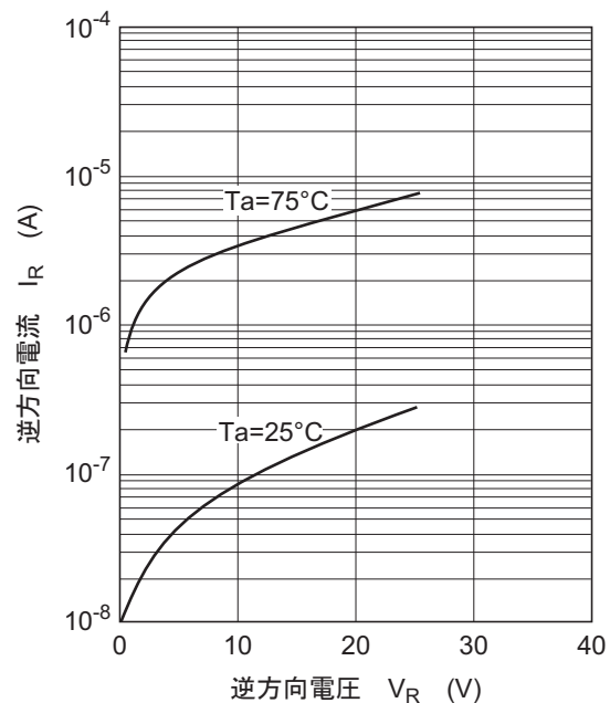
図2. 逆方向特性
