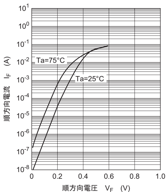
図1. 順方向特性
