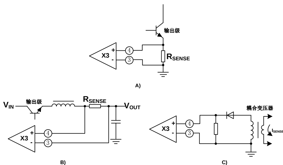
图 8-1. 峰值开关电流检测方法
