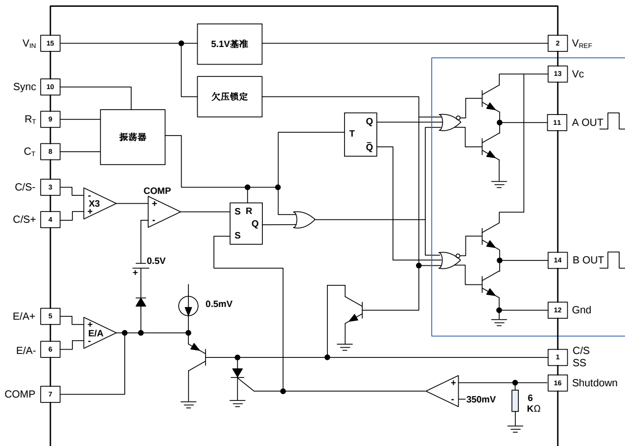
图 5-1. EG3846 结构框图
