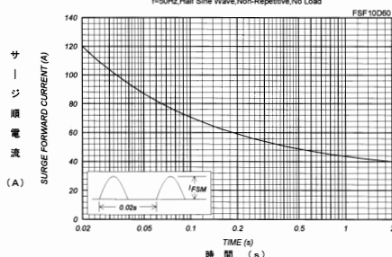
FIG.4 サーージ順電流定格 SURGE CURRENT RATINGS
