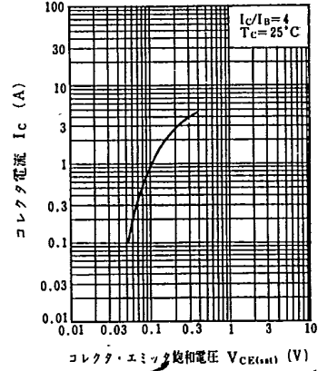
I_C - V_{CE(sat)}
