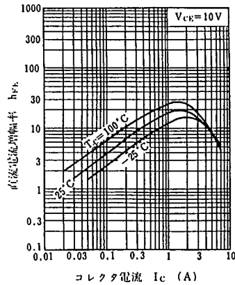
h_{FE} - I_C
